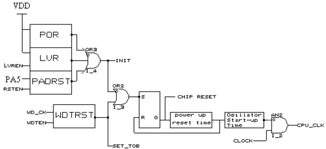
图 34 芯片复位电路框图
